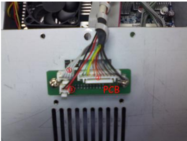
사진㉓ - 듀얼모니터 연결 케이블
